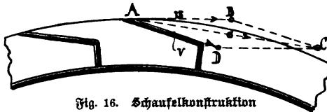
Fig. 16. Schaufelkonstruktion des ober-schlächtigen Wasserrades.
